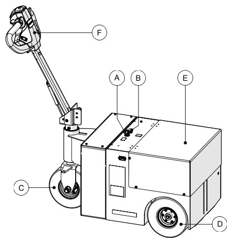
Abbildung 1. Produktübersicht
