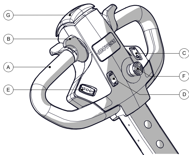
Abbildung 2. Übersicht Deichselkopf
