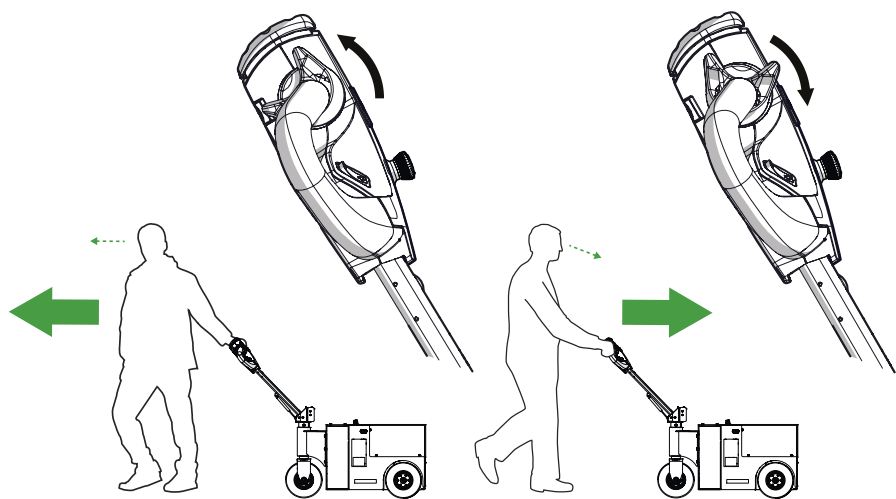
Abbildung 8. Antriebssteuerungshebel (DCL)
