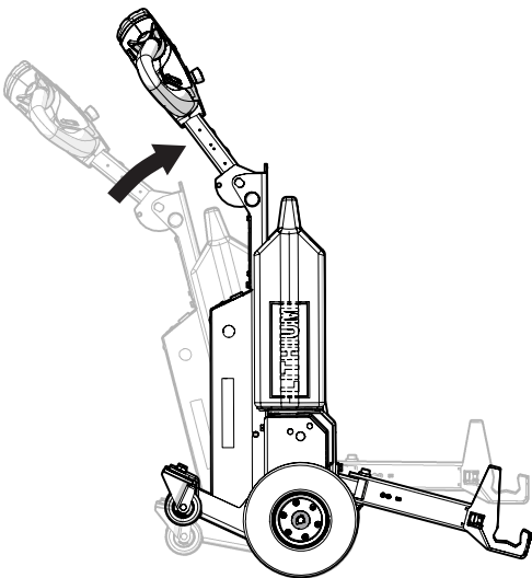
Abbildung 10. Absenken des Hakens
