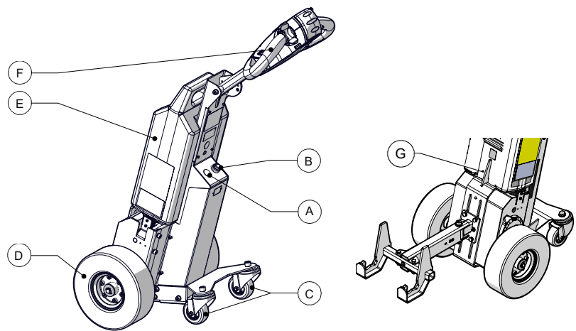
Abbildung 1. Produktübersicht
