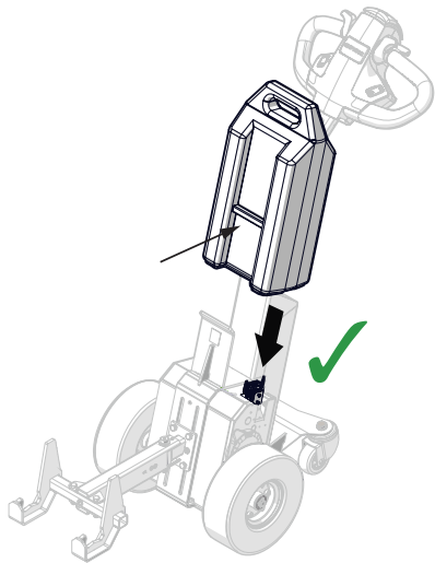
Abbildung 15. Akku einsetzen
