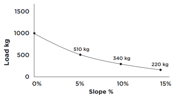
Abbildung 19. Maschinenkapazität
