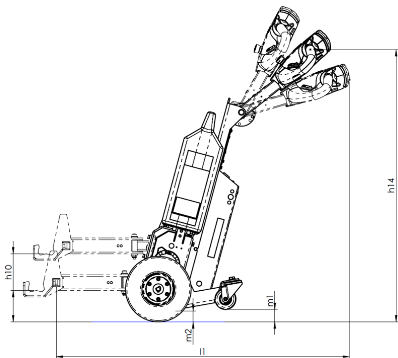
Abbildung 21. Produktabmessungen (Seitenansicht)
