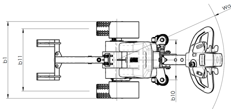
Abbildung 20. Produktabmessungen (Ansicht von oben)
