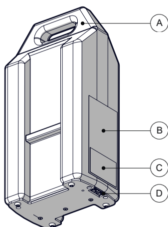
Figure 13. Vue d'ensemble de la batterie
