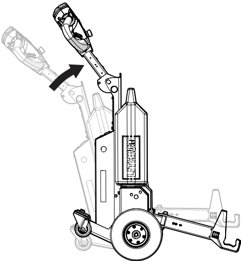
Figure 10. Abaisser le crochet
