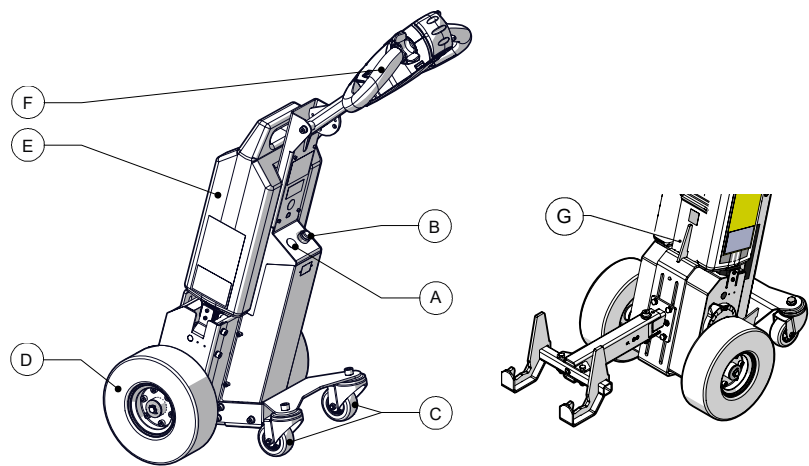
Figure 1. Vue d'ensemble du produit
