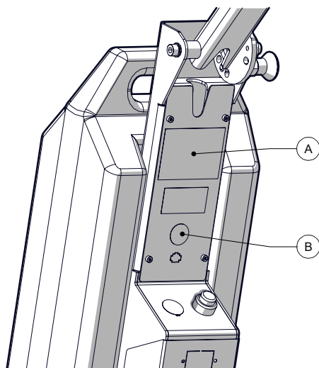
Figure 3. Identification du produit
