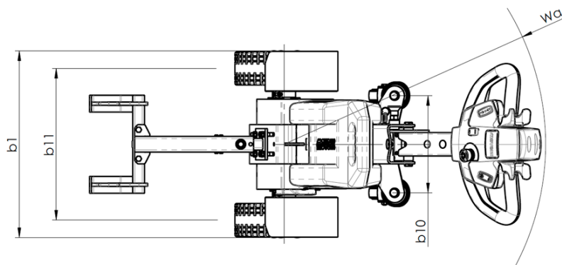
Figure 20. Dimensions du produit (vue de dessus)
