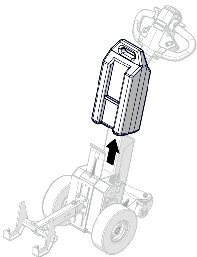
Figure 14. Retirer la batterie
