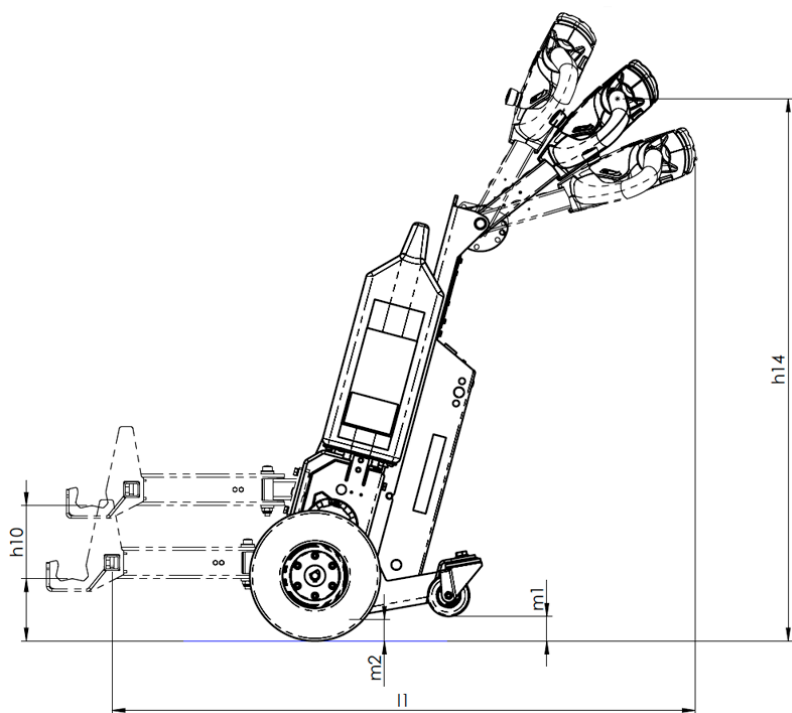
Figure 21. Dimensions du produit (vue latérale)
