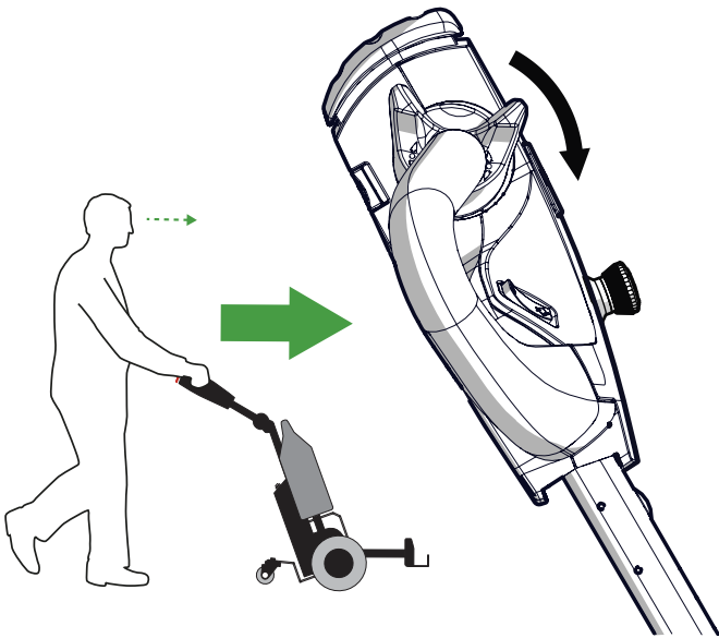
Figure 8. Levier de commande de l'entraînement (DCL)
