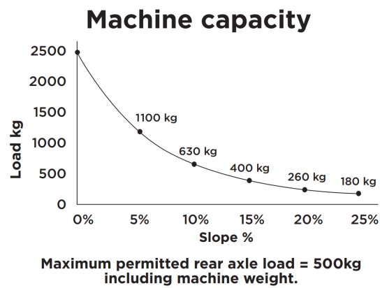
Abbildung 16. Maschinenkapazität
