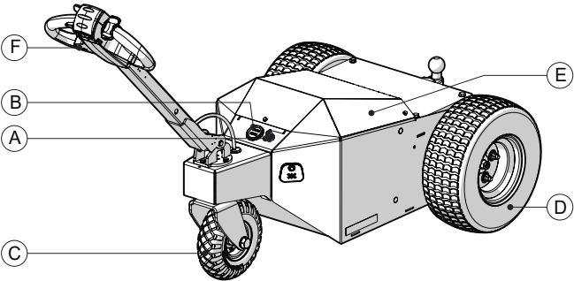
Abbildung 1. Produktübersicht
