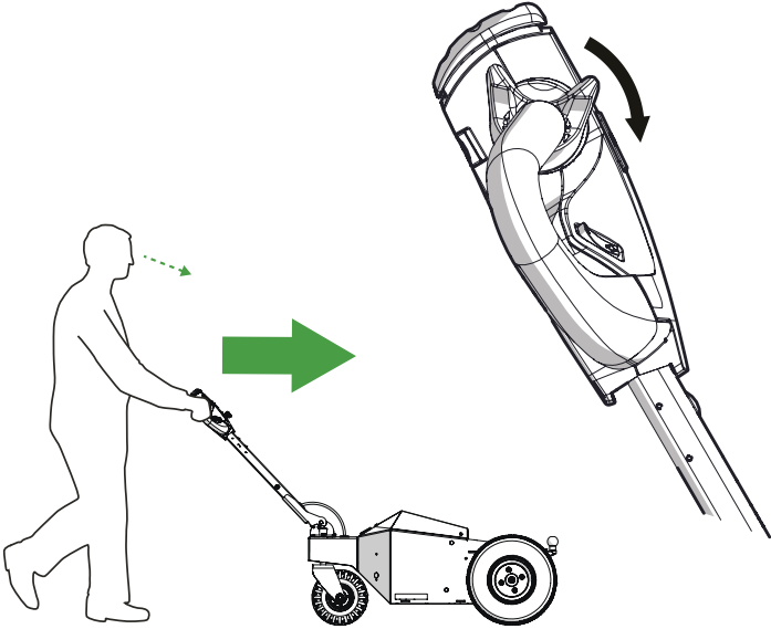
Abbildung 9. Antriebssteuerungshebel (DCL)
