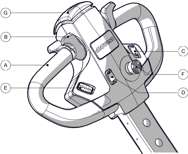
Abbildung 2. Übersicht Deichselkopf
