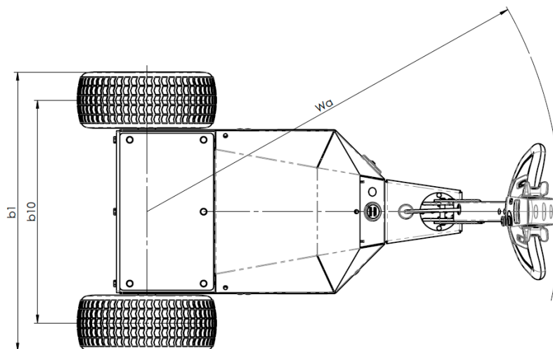
Abbildung 17. Produktabmessungen (Ansicht von oben)
