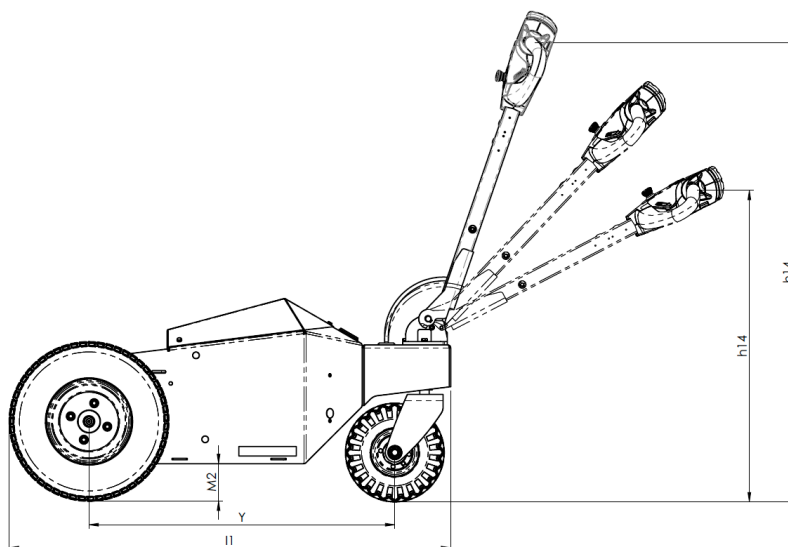
Abbildung 18. Produktabmessungen (Seitenansicht)
