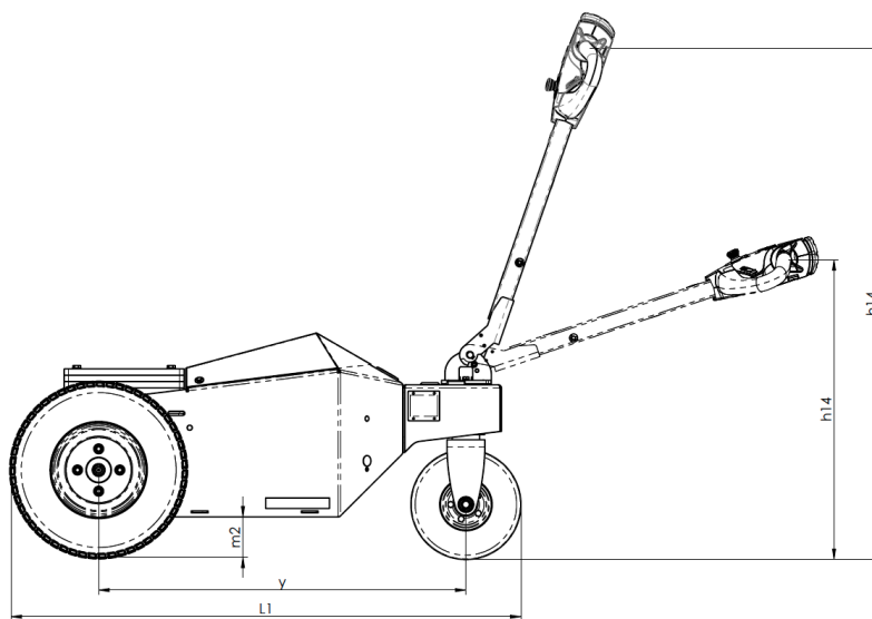
Abbildung 18. Produktabmessungen (Seitenansicht)
