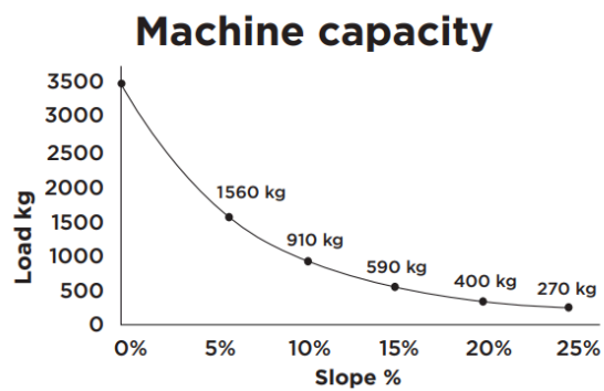
Abbildung 16. Maschinenkapazität
