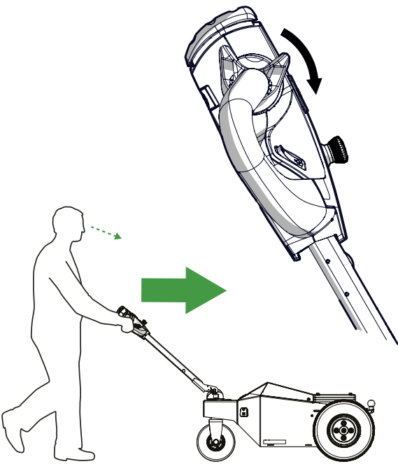
Abbildung 9. Antriebssteuerungshebel (DCL)
