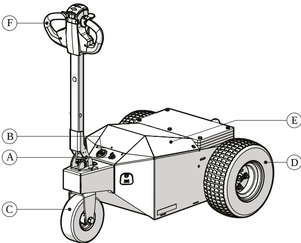
Abbildung 1. Produktübersicht
