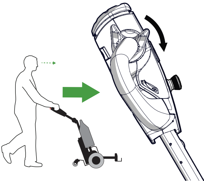
Abbildung 8. Antriebssteuerungshebel (DCL)
