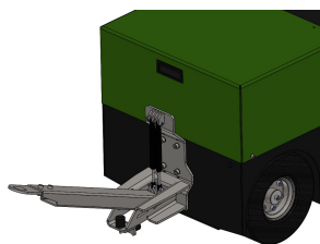
Artikel H0128-D27 Klapphaken Ø27
