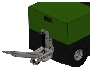
Artikel H0128-D35 Klapphaken Ø35
