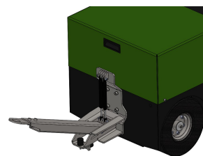
Artikel H0128-D32 Klapphaken Ø32
