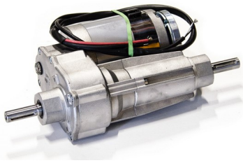
Artikel M1033-SP Motor 300W / 100 U/min, mit Bremse
