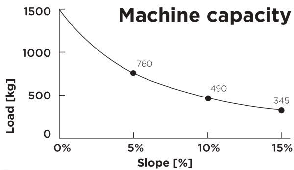
Figure 19. Capacité de la machine
