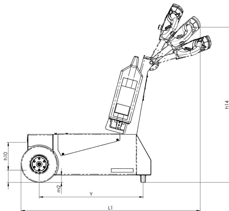
Figure 21. Dimensions du produit (vue latérale)
