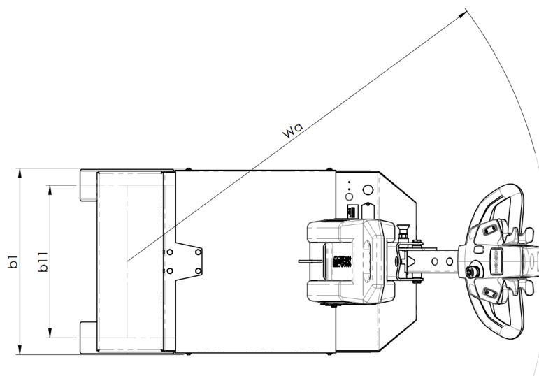
Figure 20. Dimensions du produit (vue de dessus)
