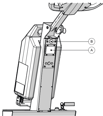
Figure 3. Identification du produit
