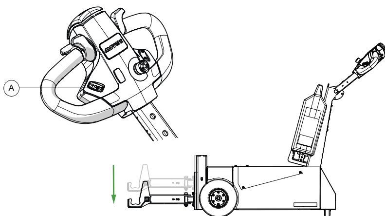
Figure 10. Abaisser le crochet
