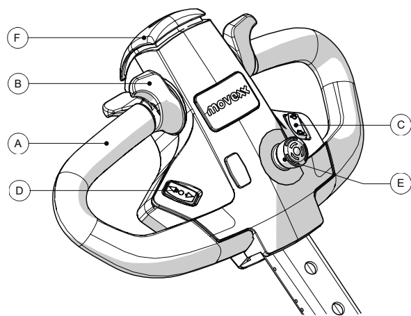
Figure 2. Vue d'ensemble de la tête de timon
