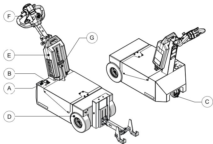
Figure 1. Vue d'ensemble du produit
