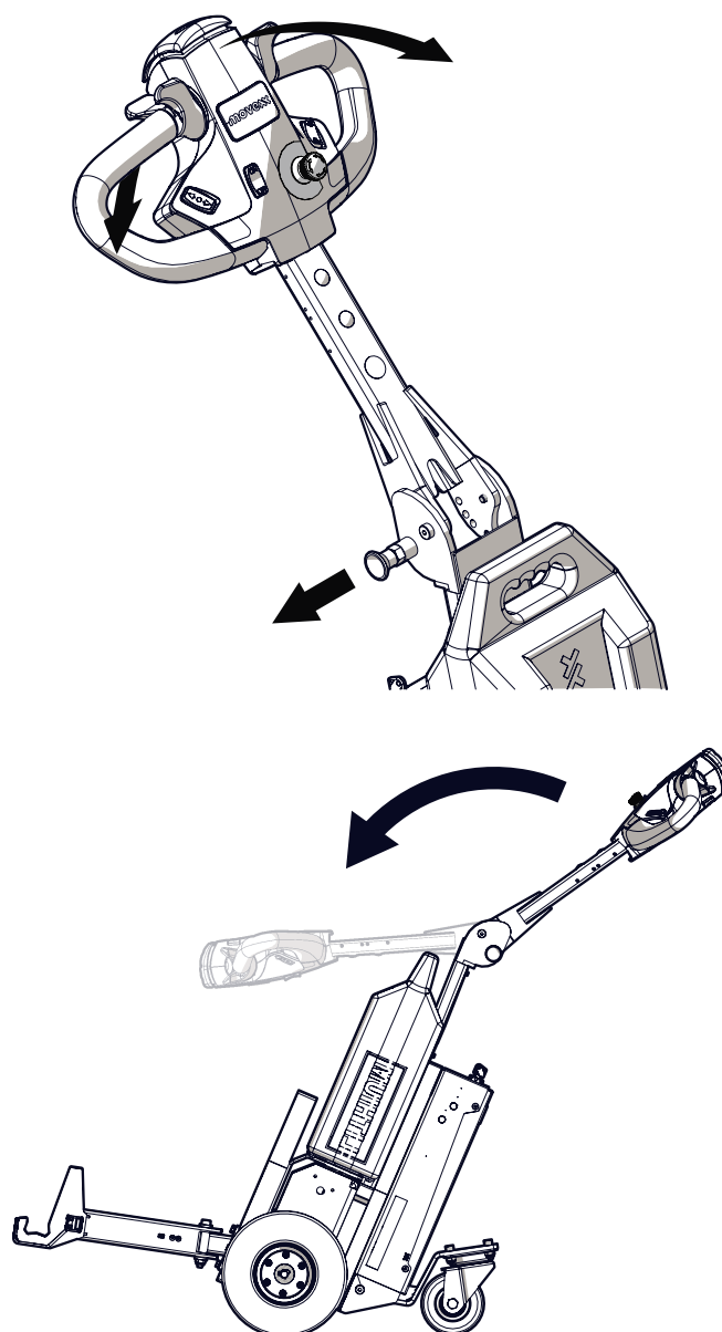
Abbildung 8. Höhe des Deichselkopfes
