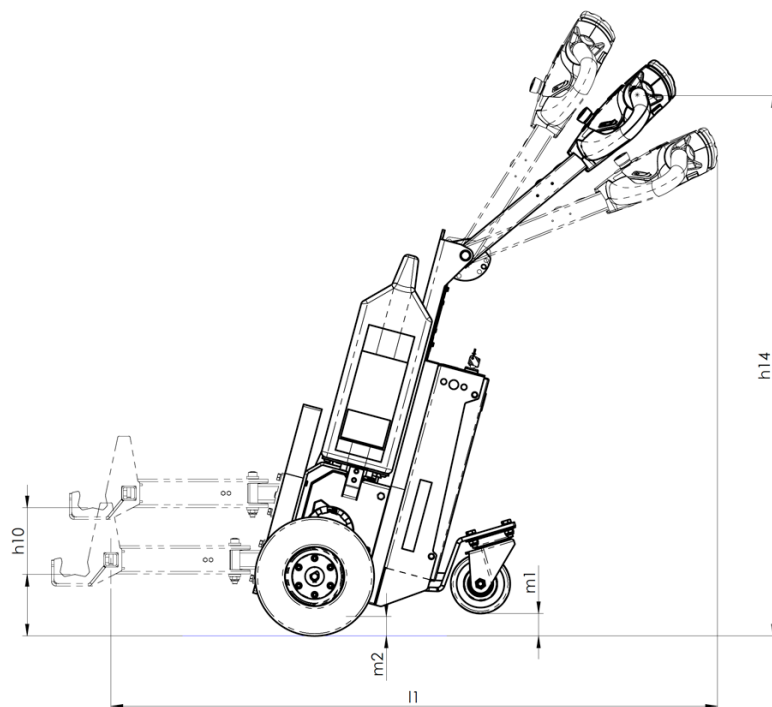
Abbildung 22. Produktabmessungen (Seitenansicht)
