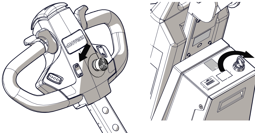
Abbildung 5. Einschalten des Produkts
