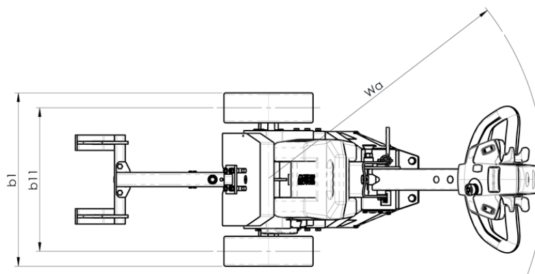
Abbildung 21. Produktabmessungen (Ansicht von oben)
