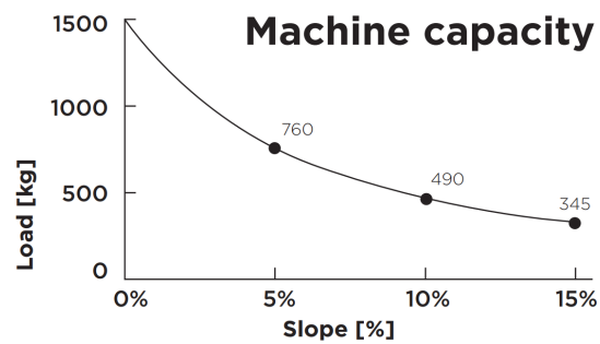
Abbildung 20. Maschinenkapazität
