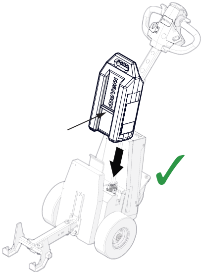
Abbildung 16. Akku einsetzen
