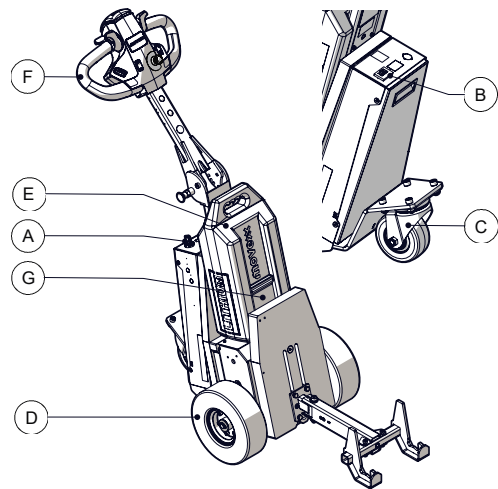
Abbildung 1. Produktübersicht
