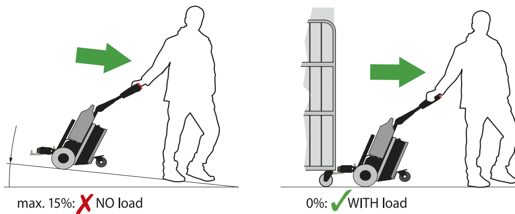
Abbildung 7. Fahren an Abhängen. Geringere Belastung an Hängen. Siehe Tabelle Maschinenkapazität.
