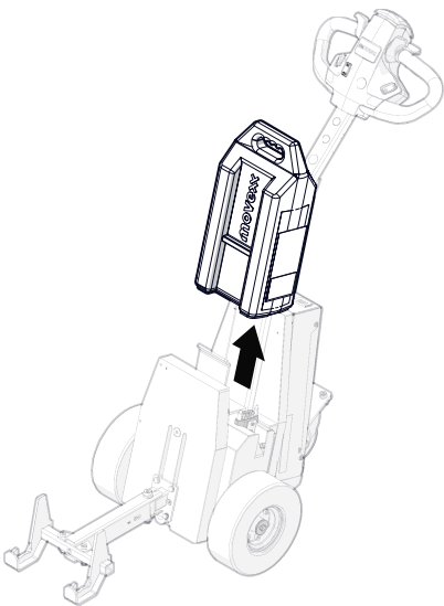
Abbildung 15. Akku entfernen
