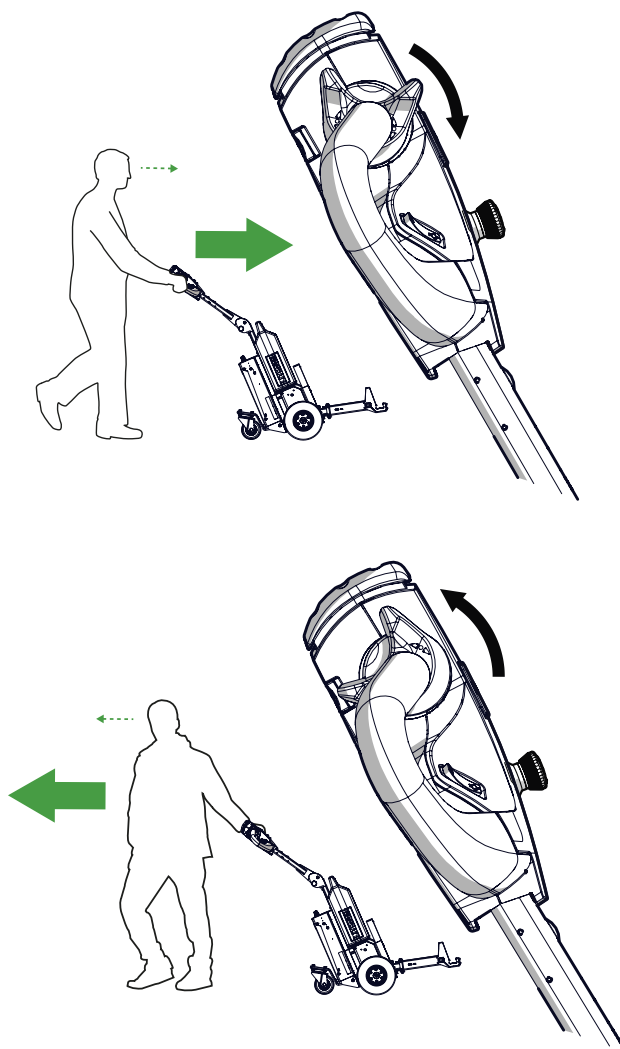
Abbildung 9. Antriebssteuerungshebel (DCL)
