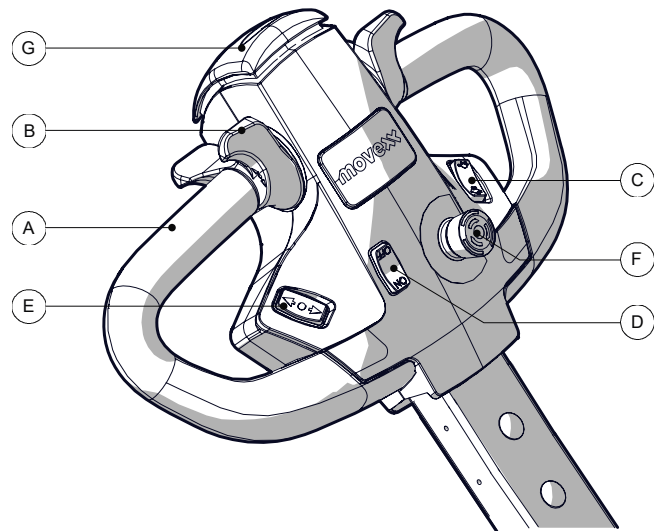
Abbildung 2. Übersicht Deichselkopf
