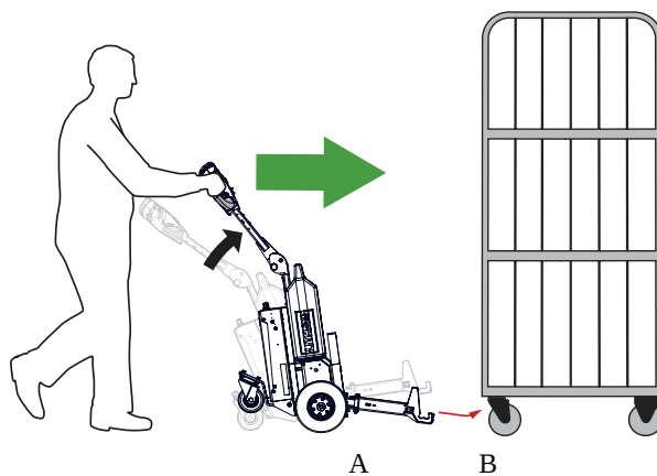
Abbildung 11. Absenken des Hakens
