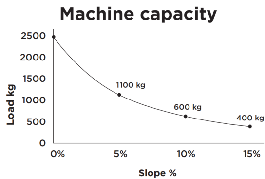
Abbildung 16. Maschinenkapazität
