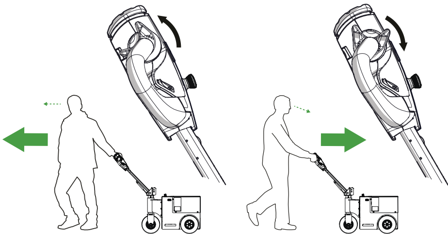
Abbildung 8. Antriebssteuerungshebel (DCL)
