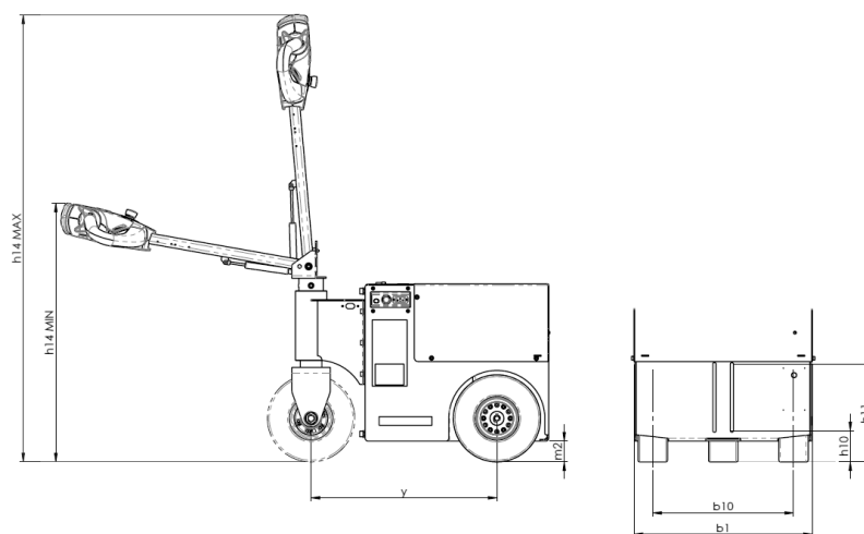
Abbildung 18. Produktabmessungen (Seitenansicht)
