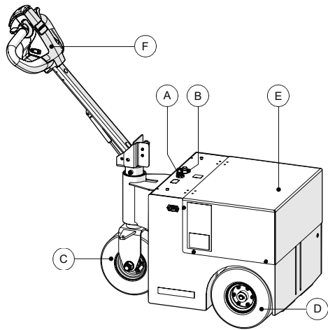
Abbildung 1. Produktübersicht
