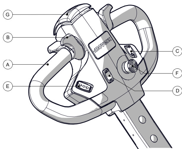
Abbildung 2. Übersicht Deichselkopf
