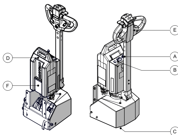
Abbildung 2. Übersicht über die Antriebseinheit
