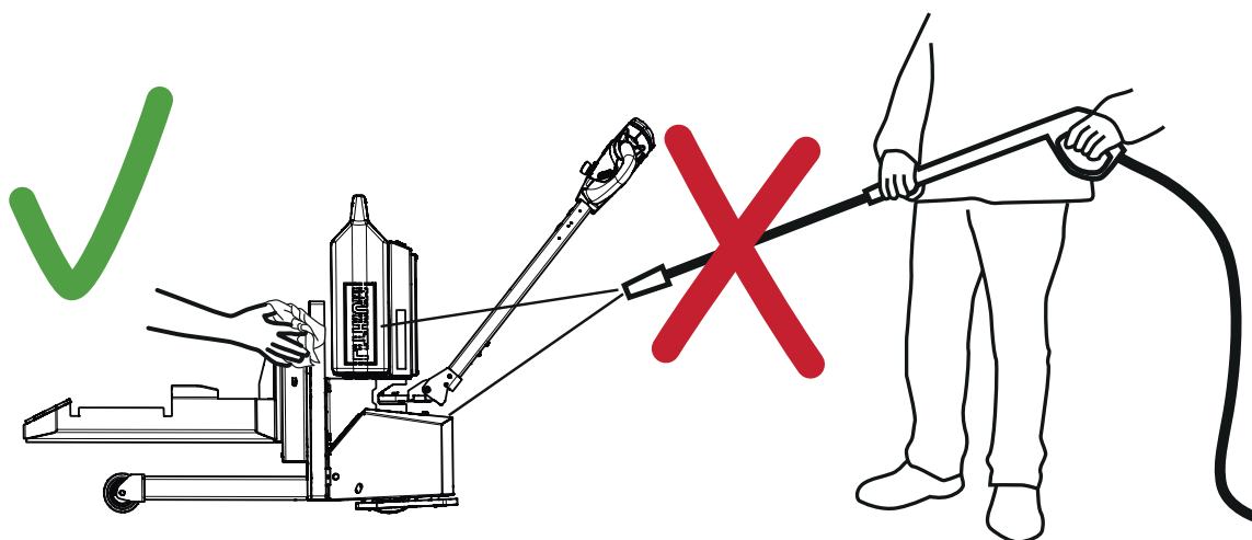
Abbildung 20. Reinigung des Produkts
