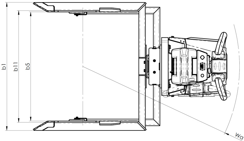
Figure 22. Produktabmessungen (Ansicht von oben)
