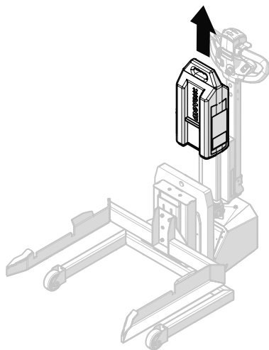
Abbildung 16. Akku entfernen
