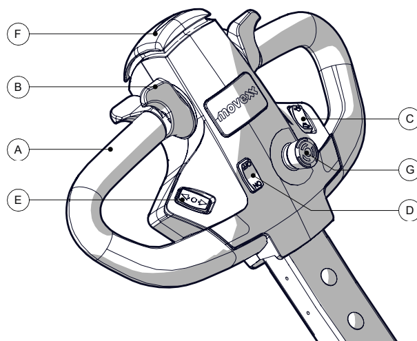
Abbildung 3. Übersicht Deichselkopf
