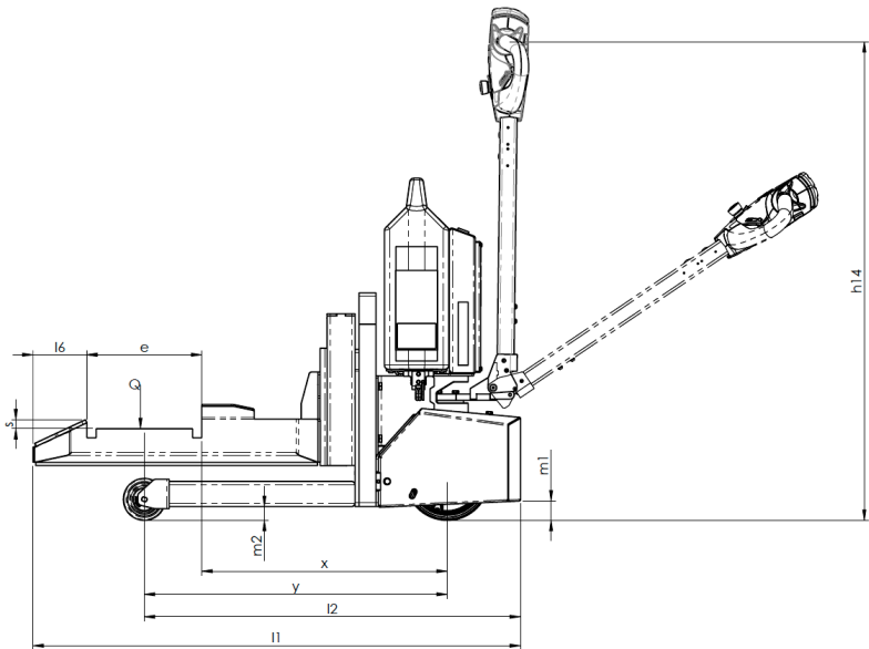
Figure 23. Produktabmessungen (Seitenansicht)
