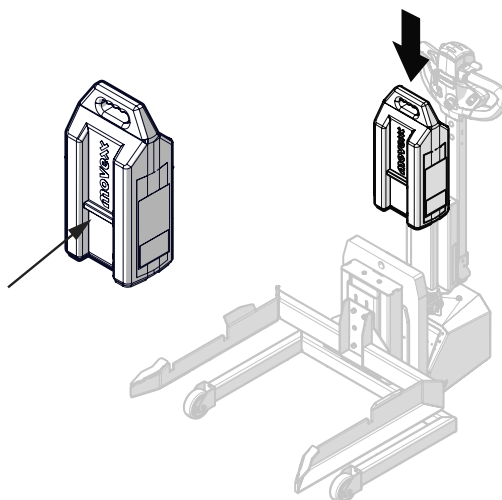
Abbildung 17. Akku einsetzen
