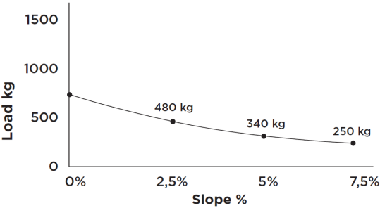
Figure 21. Maschinenkapazität
