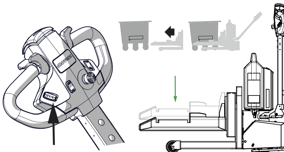
Abbildung 12. Absenken des Hakens
