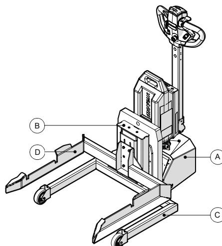
Abbildung 1. Produktübersicht
